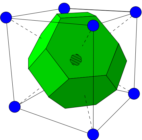
Wigner-Seitz Cell
